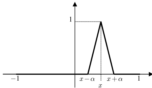
FIGURE 1 – La fonction f
