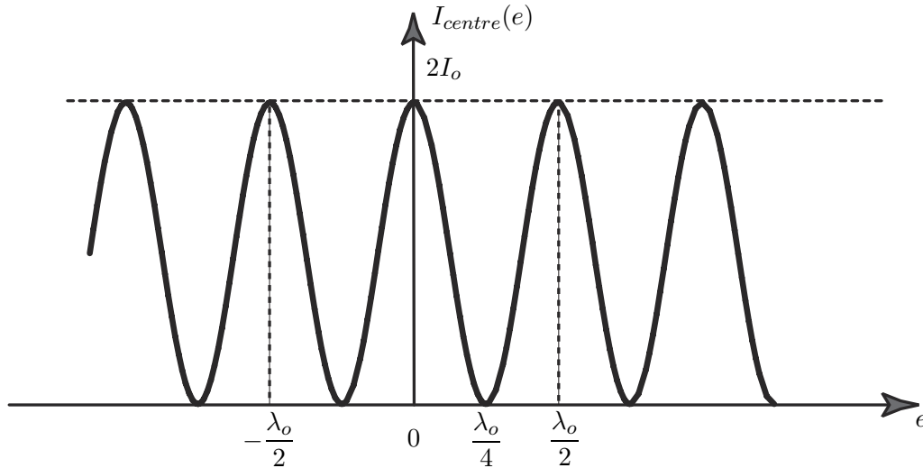
Figure 7 Intensité lumineuse au centre de la figure d'interférences I_{\text{centre}}(e)
