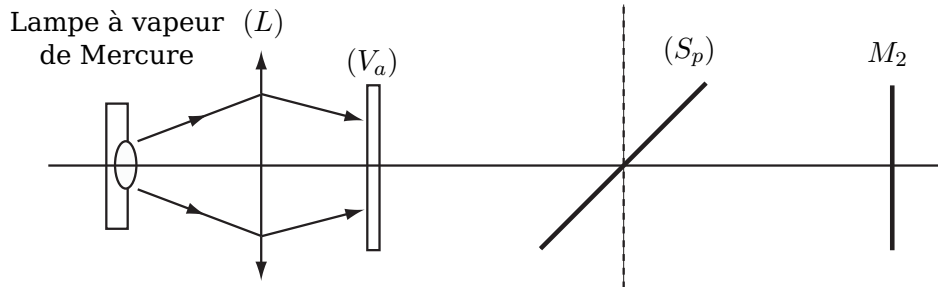
Figure 4 L'interféromètre (de Michelson) éclairé par une lampe à vapeur de mercure
