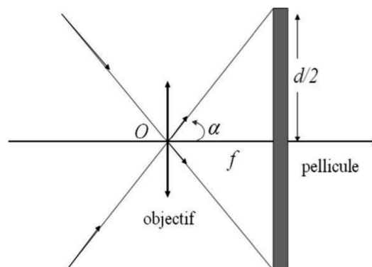
Figure 3 : champ angulaire
