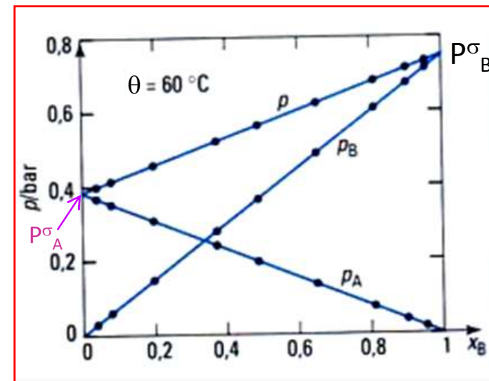
Mélange binaire idéal triéthylènamine (A) – hexane (B) : P = P_A + P_B , P_A et P_B en fonction de x_B
