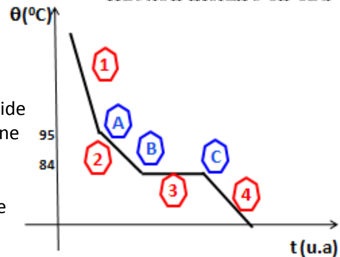
courbe de refroidissement pour le mélange de vapeur de composition y_e = 0,3
