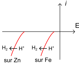
influence de la nature de l'électrode
